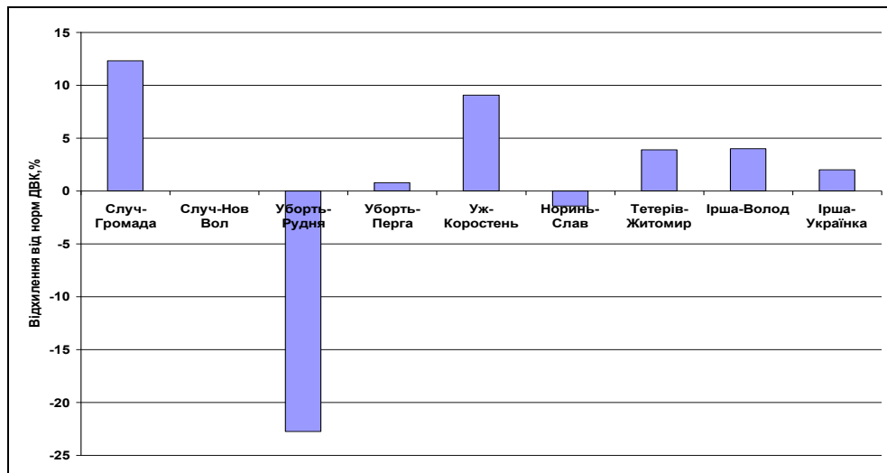
Рис. 3.4 Відхилення (%) норм водності отриманих з урахуванням циклічності від офіційних розрахункових норм ДВК, 2005 р.
