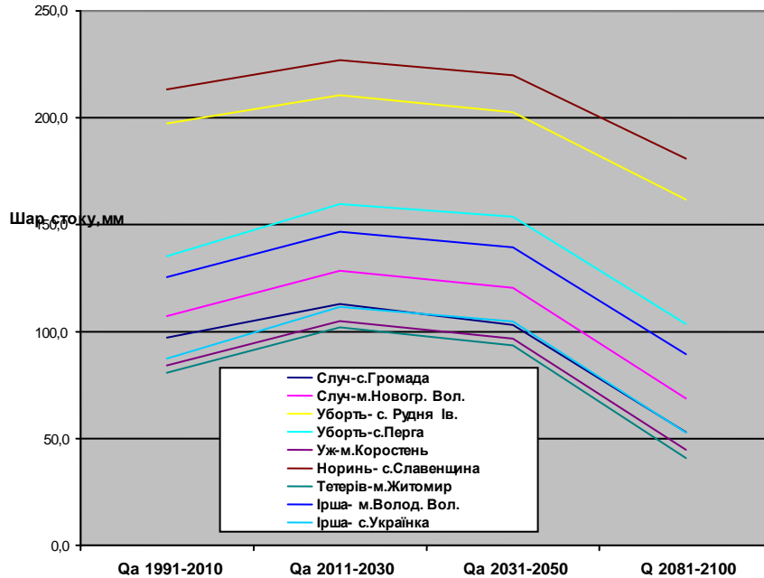
Рис. 5.4 Прогноз шару водного стоку з урахуванням середніх прогнозних величин кліматичних показників
