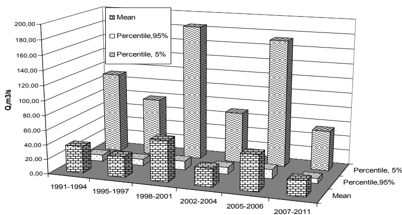
Рис. 3.18 Порівняння розрахованих характерних витрат води за виділені періоди
