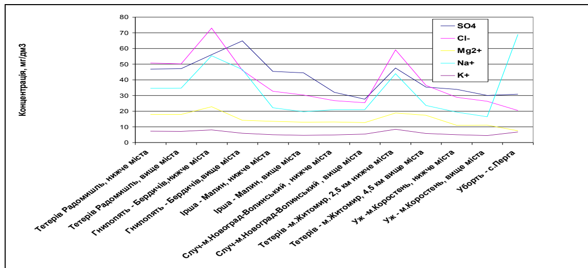
Рис. 4.4 Середні концентрації другорядних за величинами концентрацій аніонів та катіонів розчинених у воді солей SO_4^{2-} , Cl^- , Mg^{2+} , Na^+
