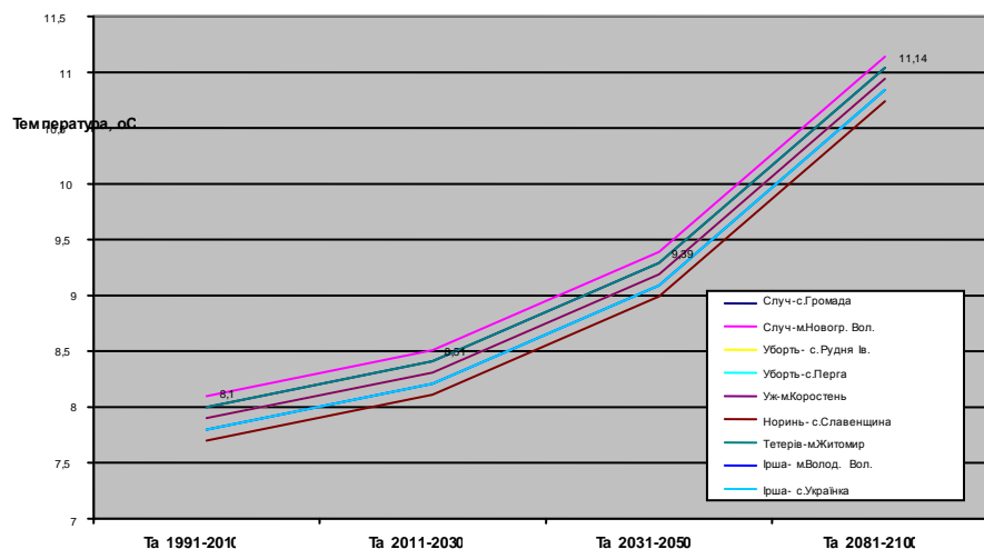
Рис. 5.1 Зміна середніх річних величин температури протягом ХХІ століття в межах досліджуваних водозбірних басейнів
