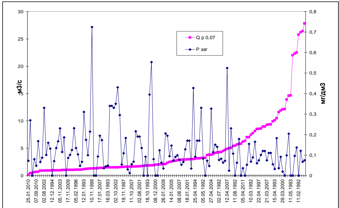
Рис. 4.16 Співставлений графік ранжованих вимірних витрат води р.Уж в створі нижче м.Коростеня з відповідними їм концентраціями Р заг.
