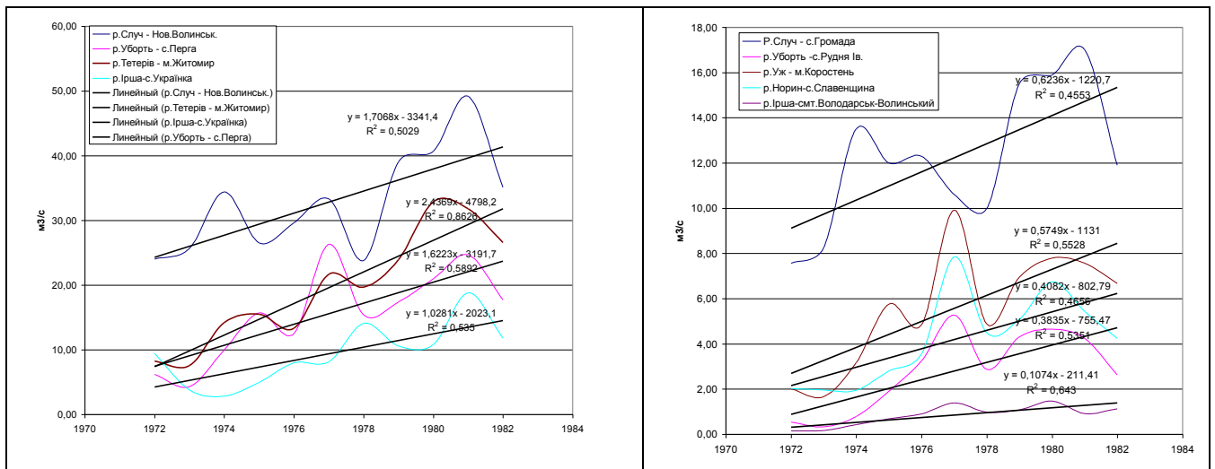
Рис. 3.7 Тренди зміни водного стоку протягом 1972-1982 рр.
