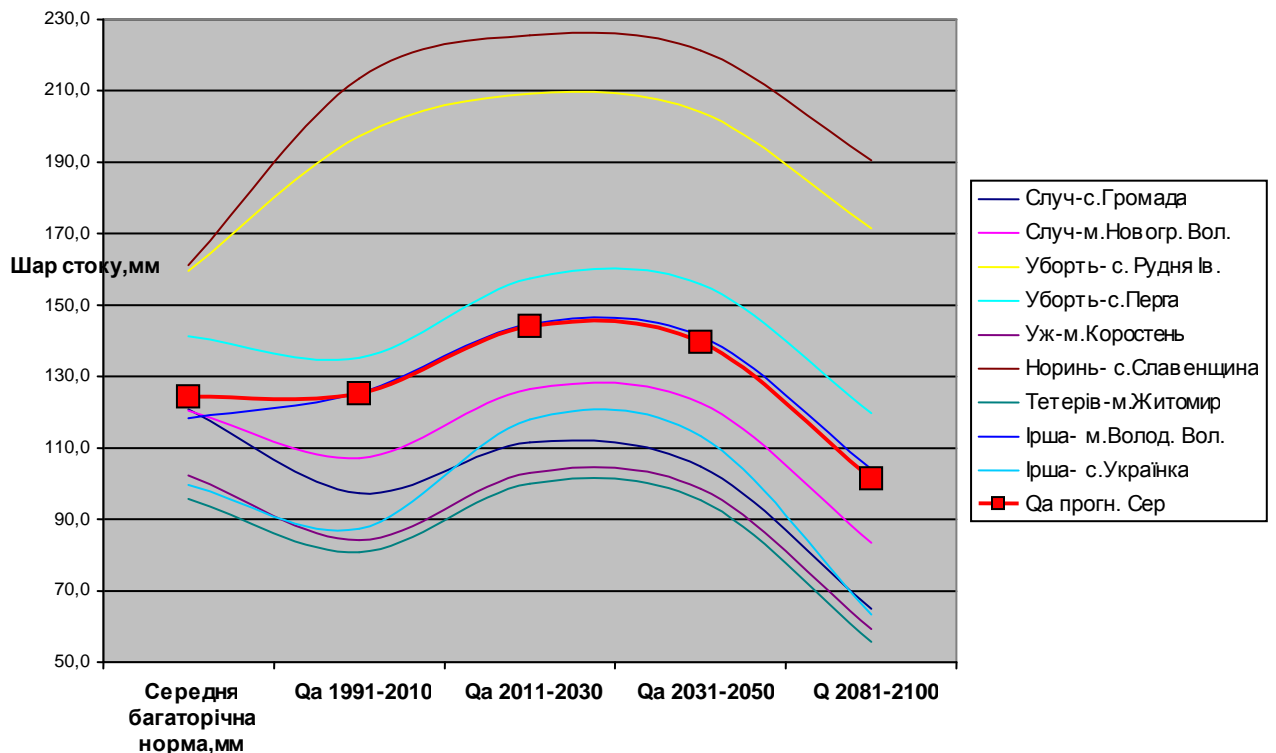
Рис. 5.7 Порівняння середніх прогнозних величин шару водного стоку по окремих річкових басейнах та середнього прогнозного шару водного стоку території Житомирського Полісся з середніми багаторічними нормами водного стоку
