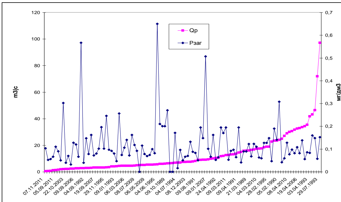
Рис. 4.17 Співставлений графік ранжованих вимірних витрат води р.Уборть в створі с. Перга з відповідними їм концентраціями Р заг.
